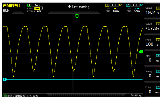
Gambar 3.10 Hasil Output Penyearah
